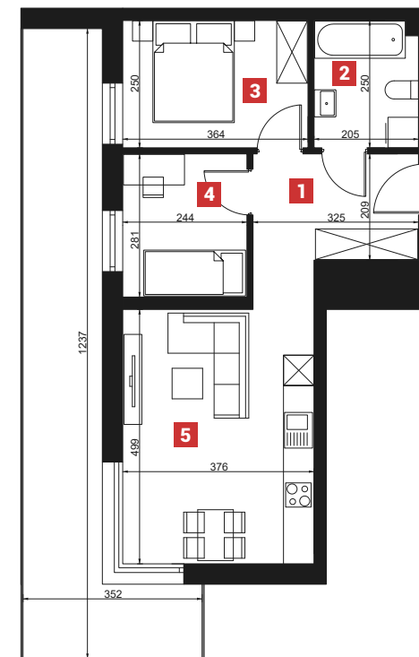
Rzut mieszkania M7
