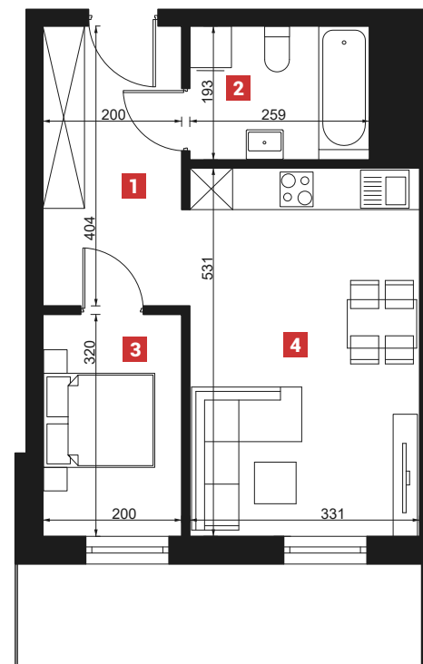
Rzut mieszkania M31
