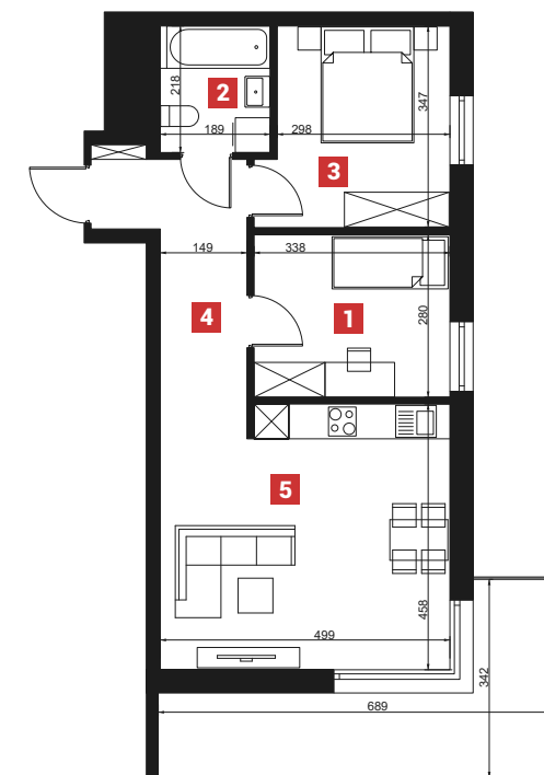
Rzut mieszkania M30
