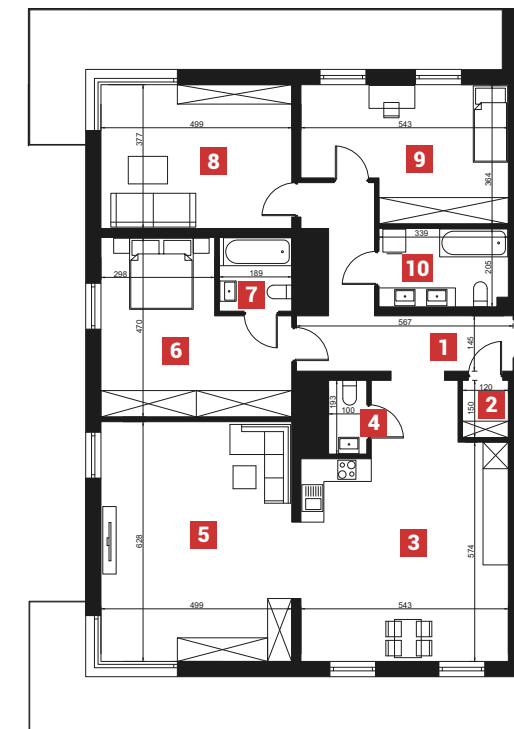
Rzut mieszkania M44
